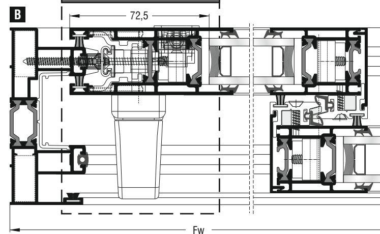
Κλειδαριά BEZAUPT RIVALU BEZAUPT RIVALU lock
