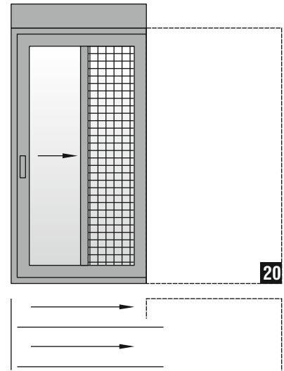
Μονόφυλλο χωνευτό συρόμενο με σήτα & ρολό One sash pocket sliding with fly-screen & rolling shutter
