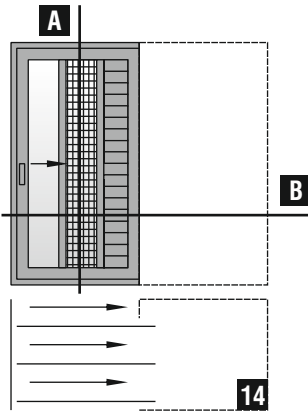
Μονόφυλλο χωνευτό συρόμενο με σήτα (φύλλο σήτας M868 ) και παντζούρι S325 One sash pocket sliding with fly-screen (M868 fly-screen sash) and shutter S325
