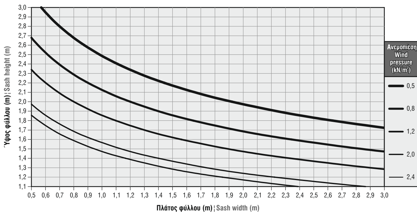
Μέγιστες διαστάσεις φύλλου για συγκεκριμένη ανεμοπίεση | Maximum sash dimensions for given wind pressure Φύλλο S384 - Μπινί S360 | S384 sash profile - S360 adjoining profile
