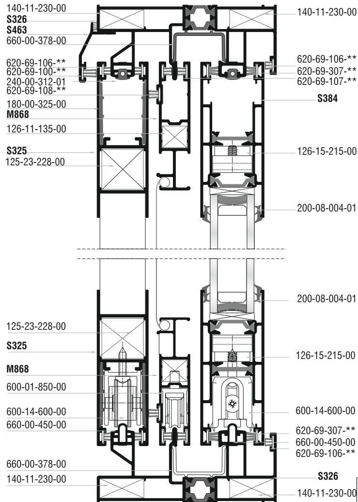
Μονόφυλλο χωνευτό συρόμενο με σήτα (φύλλο σήτας M868 ) και παντζούρι S325 One sash pocket sliding with fly-screen (M868 fly-screen sash) and shutter S325
