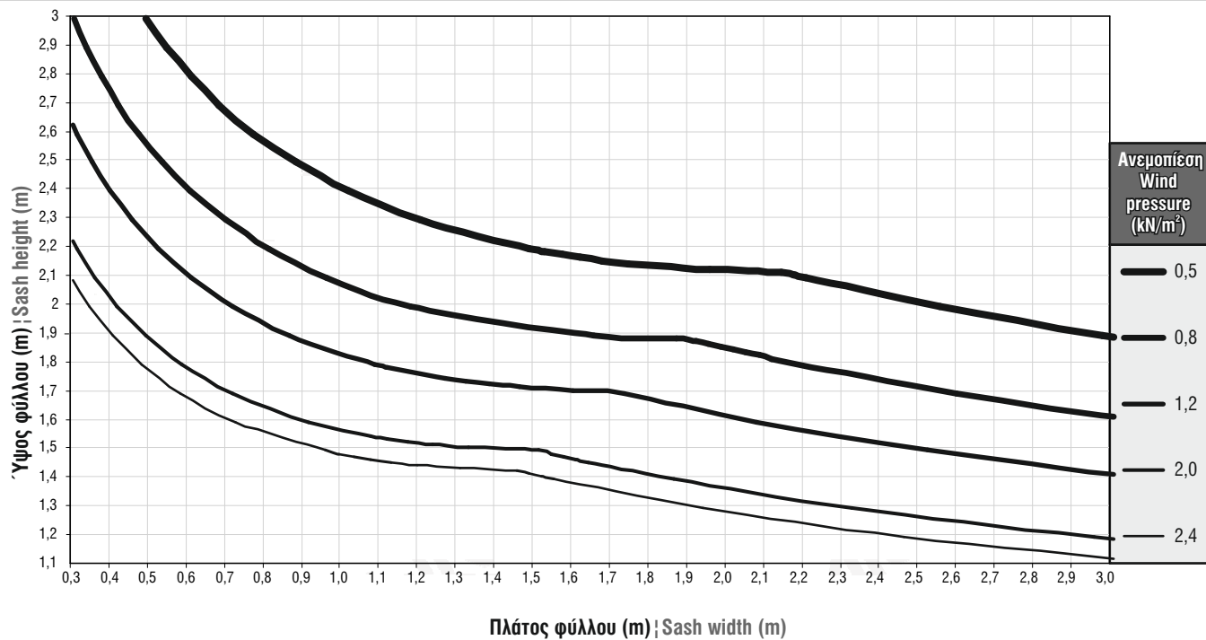
Μέγιστες διαστάσεις φύλλου για συγκεκριμένη ανεμοπίεση | Maximum sash dimensions for given wind pressure Φύλλο S384 - Άγκιστρο S362 | S384 sash profile - S362 hook profile
